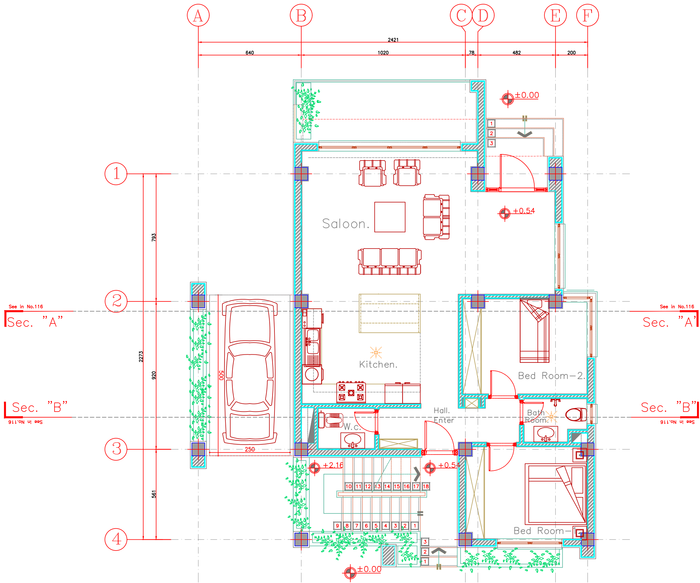
پلان مبلمان طبقه همکف Block-B Sc.1:50
